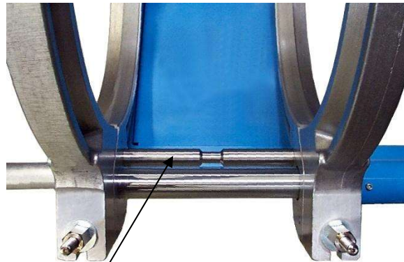
ET-Set Abreißstab komplett Grundkörper 081516KP
