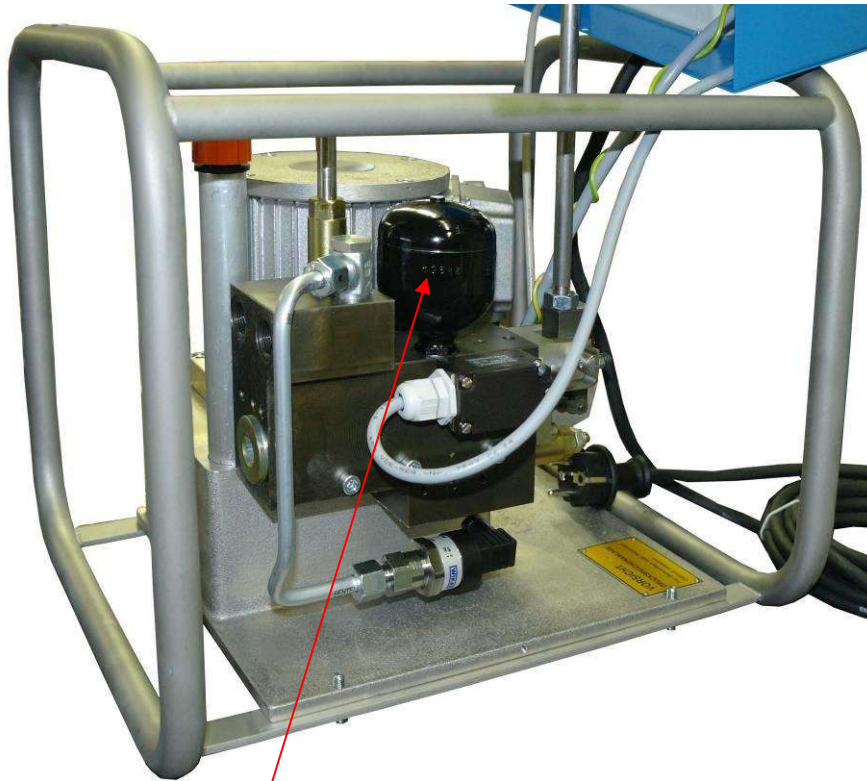
ET-Set Druckspeicher komplett Hydraulikaggregat 101006KP
