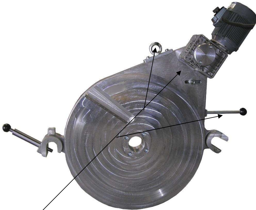
ET-Set Gehäuse Planhobelhalter komplett 0824011KP
