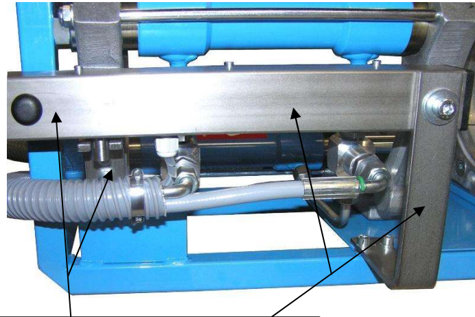
ET-Set Wegmesssystem mit / ohne Schlauch komplett 16WMSVSCHLKP / 16WMSKP
